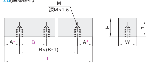
ZB(底部螺孔)
