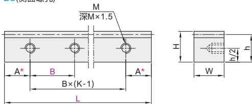
ZC(侧面螺孔)
